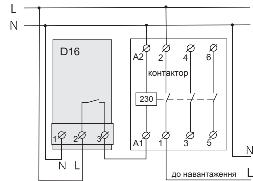
Схема 3. Підключення ZUBR D16 та контактора з обмоткою 230 В
