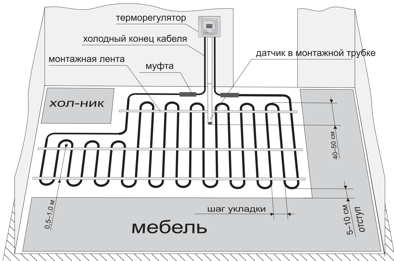
пример укладки одножильного нагревательного кабеля
